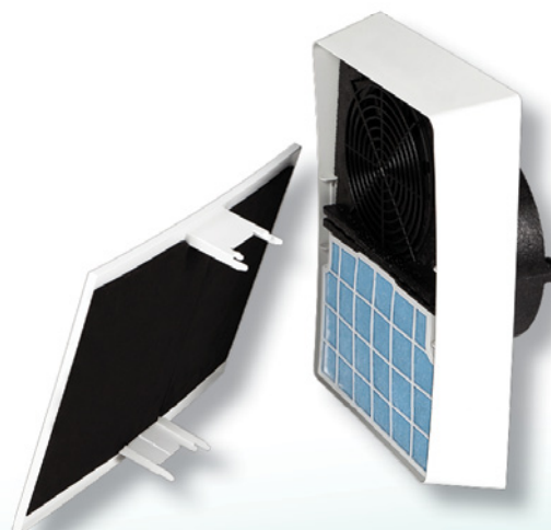
Innenblende mit Ventilatoreinheit, Luftfilter und Schalldämmeinsatz - Einfache Wartung garantiert
